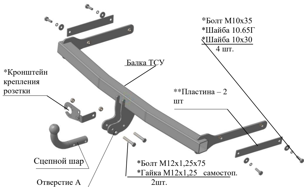
Рис.1 Тягово-сцепное устройство ТСУ 9151.
