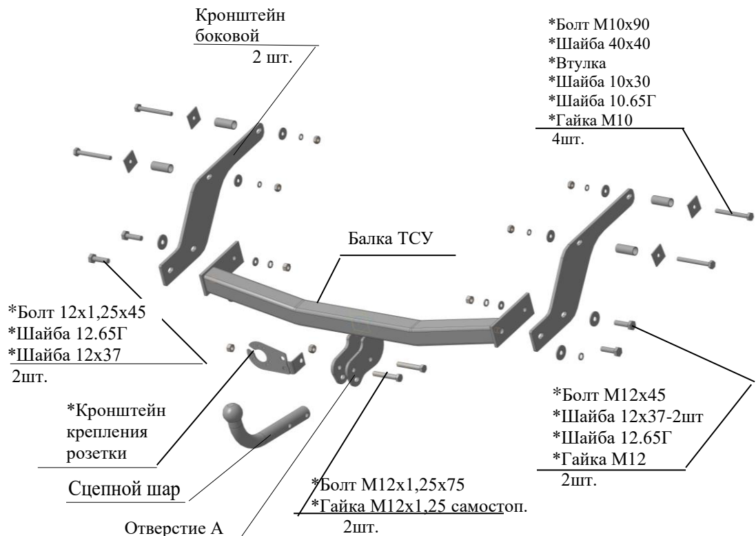
Рис.1 Тягово-сцепное устройство ТСУ 9070.
