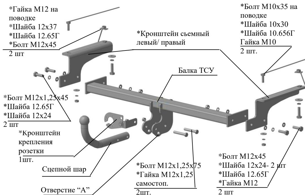
Рис.1 Тягово-цепное устройство 8140
