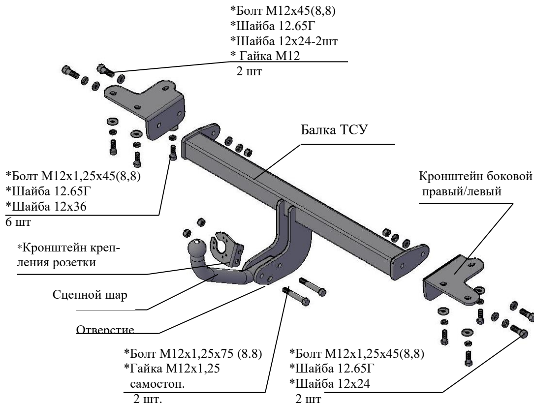
Рис.1 Тягово-сцепное устройство 7900.
