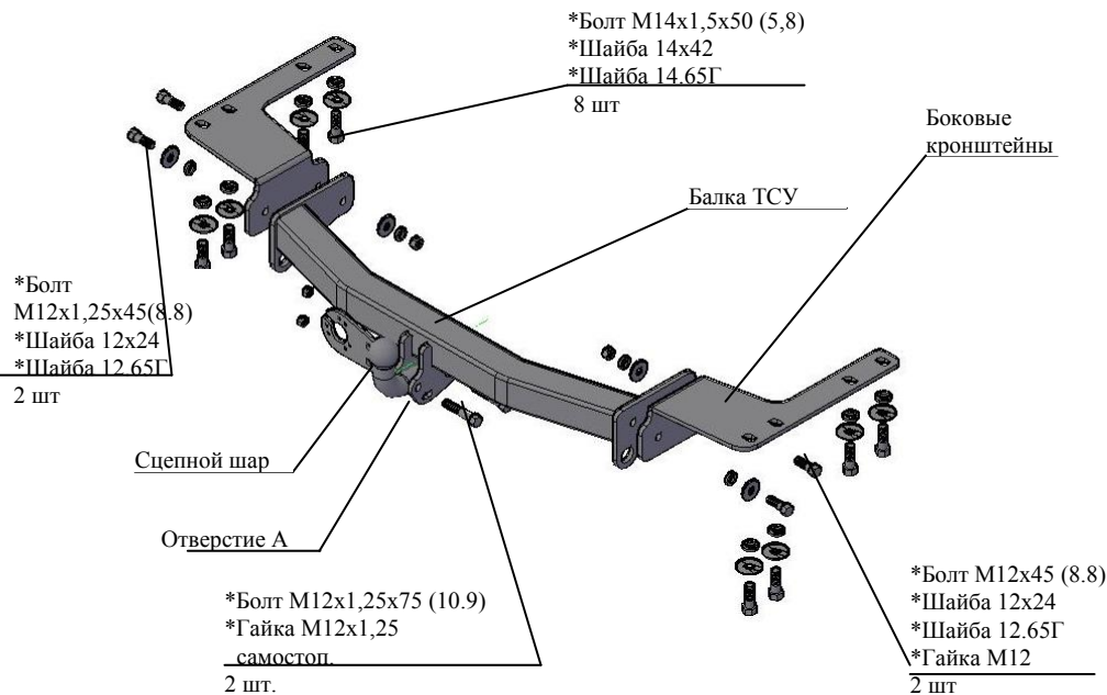
Рис.1 Тягово-сцепное устройство 7820.
